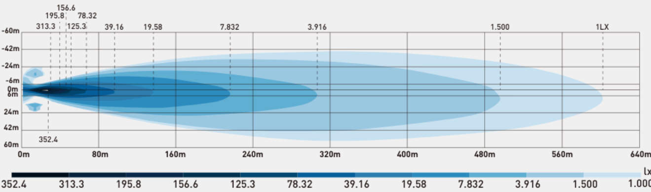
Boost : 1Lux@610m
