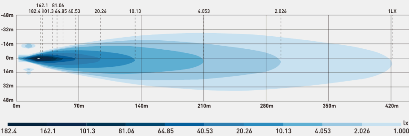
E-mode : 1lux@420m
